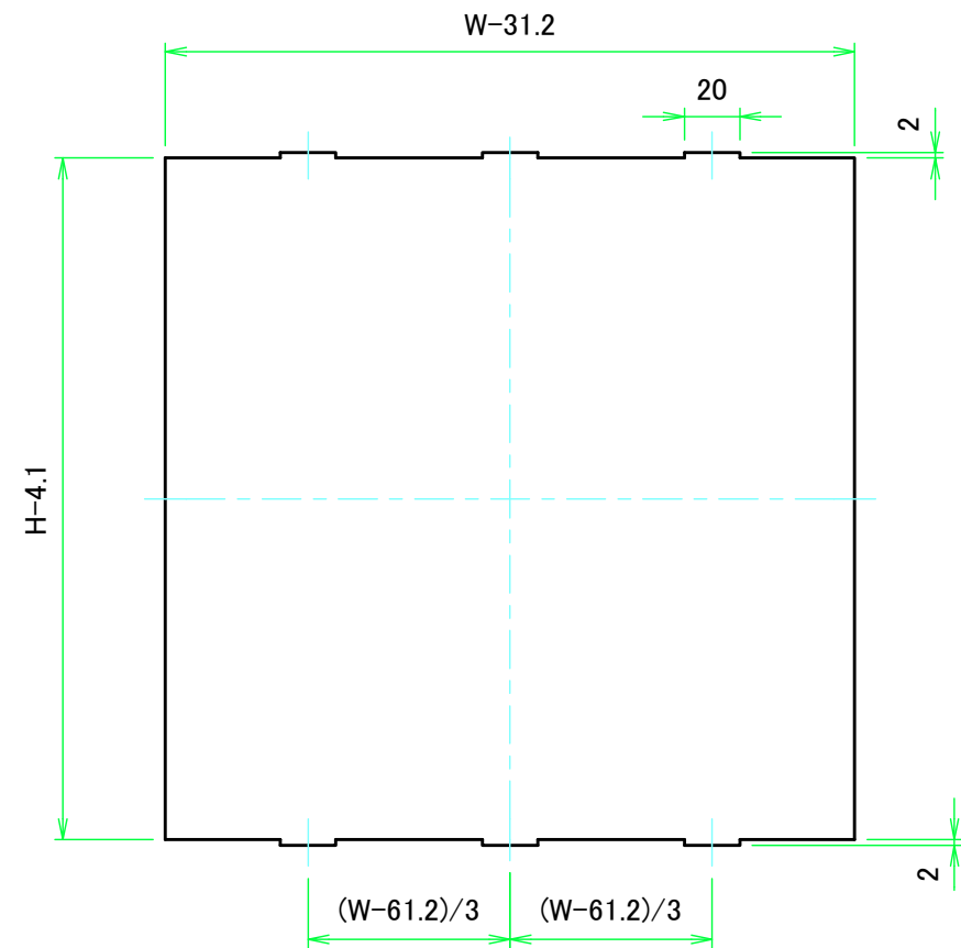
Wパネル1表面 / W Panel 1 Frontside
