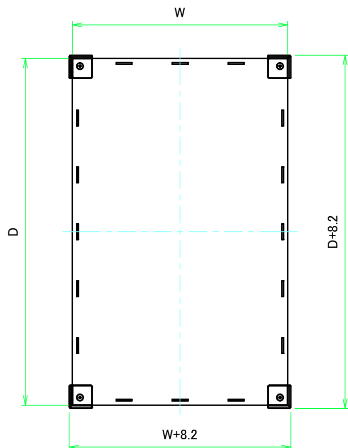
上カバー / Top cover
